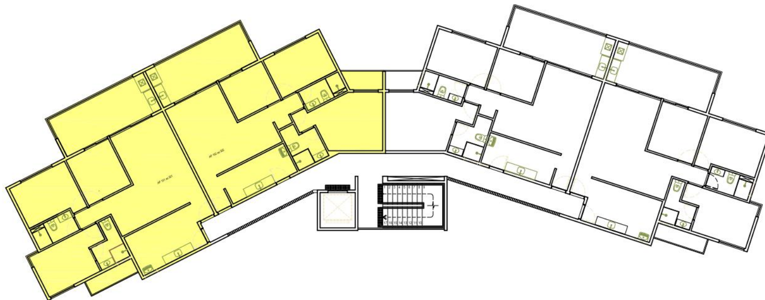
PLANTA BAIXA - TIPO 03/TORRE 03 ESCALA - 1/100
